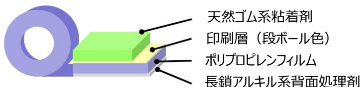
図. No.3525 テープ構成
